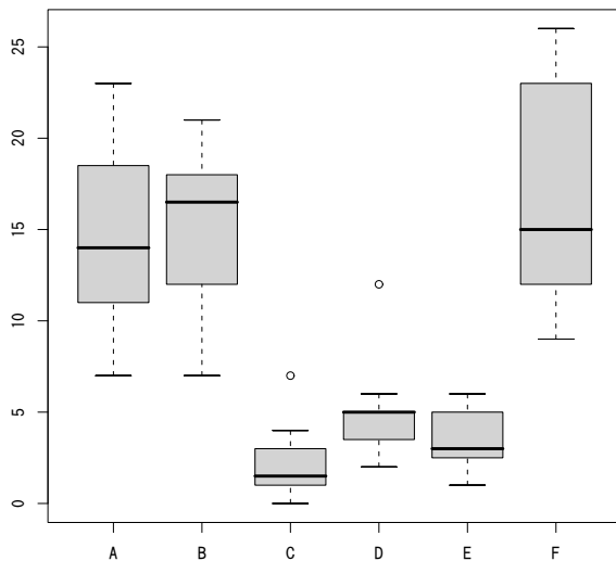
図 1: 把っ手 (notches) 付きの箱型図 (1)
