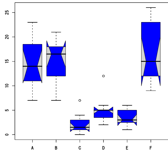
図 2: 把っ手 (notches) 付きの箱型図 (2)
